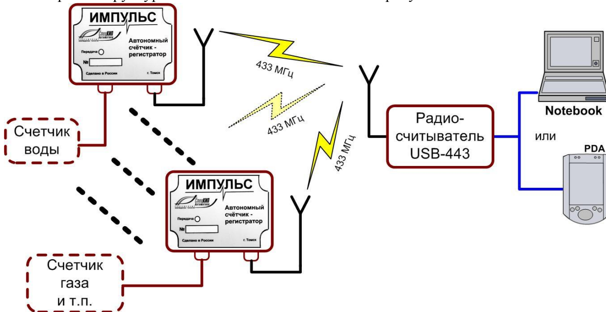
Рисунок 1 – Пример структурной схемы комплекса
