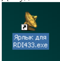
Рисунок 2 – Ярлык программы
